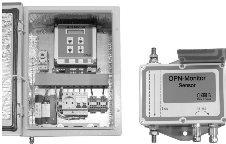
Рисунок 4 Внешний вид «ОПН-Монитора»
