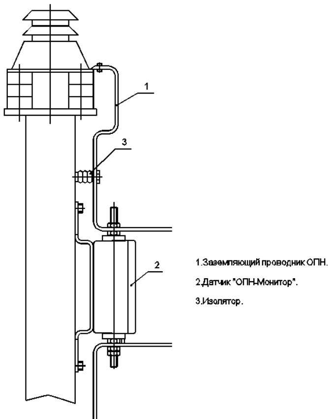
Рисунок 1 Схема включения датчика
